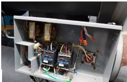
機油加熱器的供電
